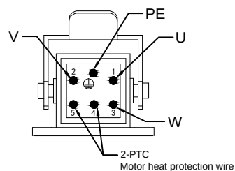
【Wiring description diagram】
